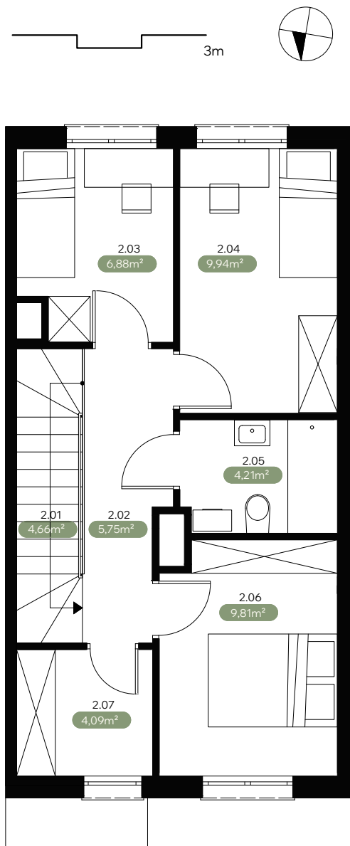
PODDASZE
